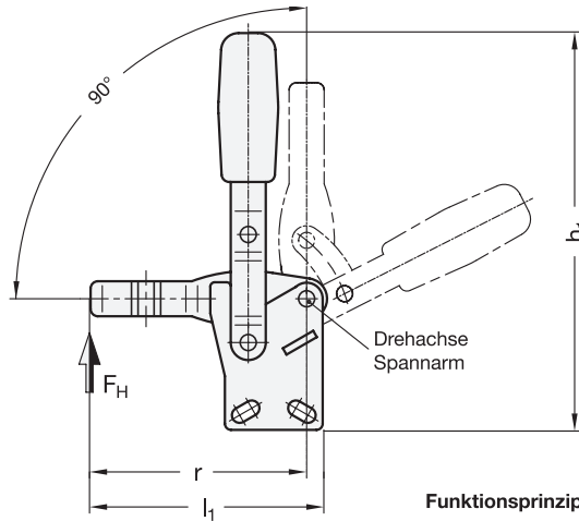
Funktionsprinzip
