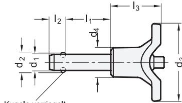
Kugeln verriegelt (90° versetzt gezeichnet)
