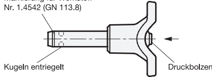
Markierung für Werkstoff Nr. 1.4542 (GN 113.8)
